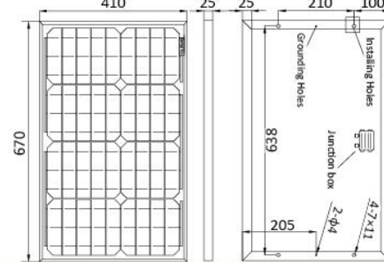
GSM-80W-M
