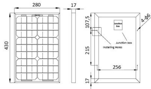
GSM-35W-M
