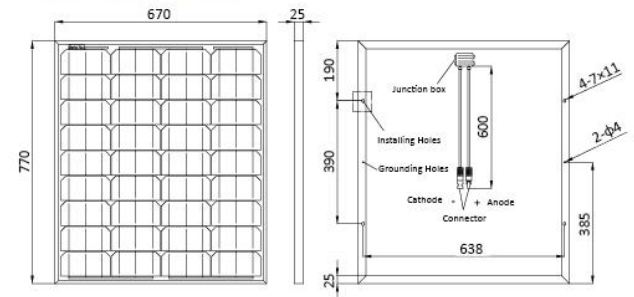
GSM-80W-M
