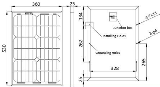
GSM-50W-M
