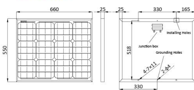
GSM-50W-M
