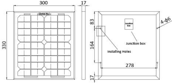
GSM-12W-M
